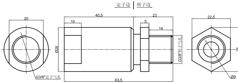
DK13A 尺寸图
