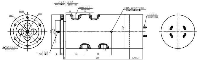
DAPH400-05 尺寸图
