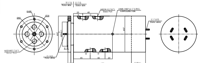
DAPH400-03 尺寸图
