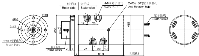
DAPH400-01 尺寸图
