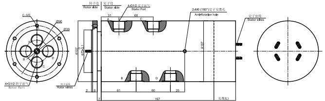
DAPH400-05 尺寸图
