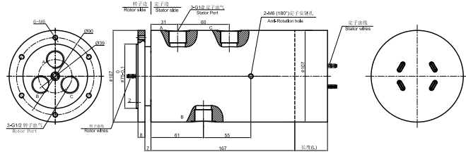
DAIPH300-05 尺寸图
