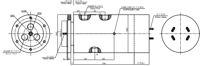
DAIPH300-04 尺寸图
