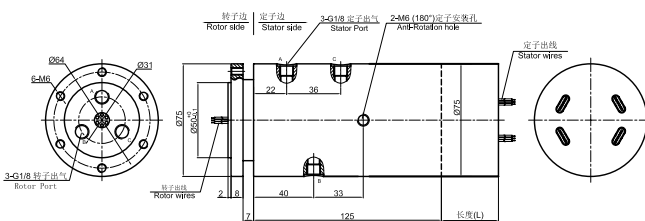
DAPH300-03 尺寸图
