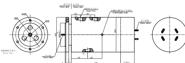
DAPH300-03 尺寸图
