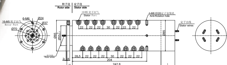
DAPH1600-01 尺寸图
