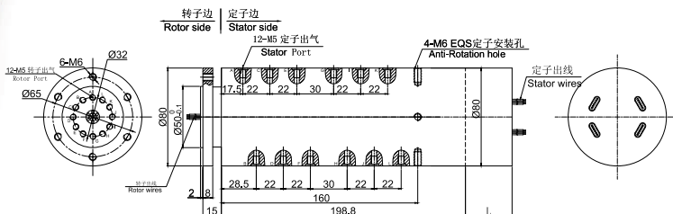
DAPH1200-01 尺寸图
