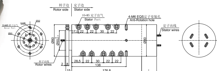
DA PH1000-01 尺寸图
